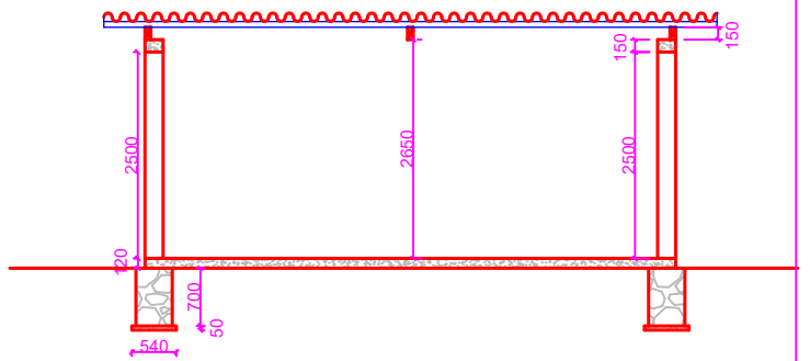
COUPE
